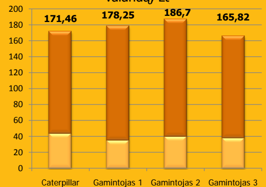
Eksplotacijos ir turėjimo kaštai per 1 moto valandą, Lt
