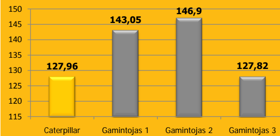
Eksplotacijos išlaidos per 1 moto valandą, Lt
