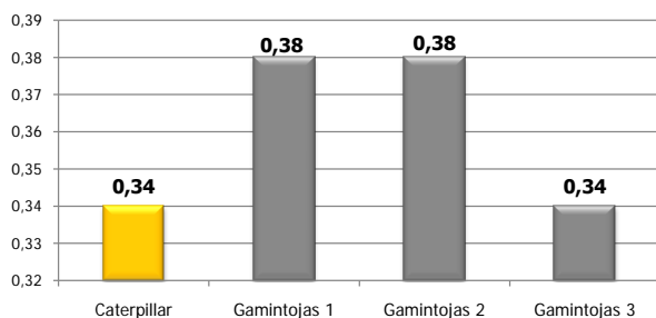
Vienos iškastos tonos savikaina, Lt
